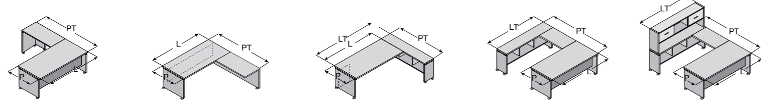
PT 190 x H 73,3 P 90 L 160 L 180 L 200 PT 190 x H 73,3 P 90 L 160 L 180 L 200 PT 200 x H 73,3 P 90 L 160 - LT 201 L 180 - LT 221 L 200 - LT 241 PT 231 x H 73,3 P 90 L 160 - LT 200 L 180 - LT 200 L 200 - LT 200 PT 231 x H 73,3 / 149,6 P 90 L 160 - LT 200 L 180 - LT 200 L 200 - LT 200
