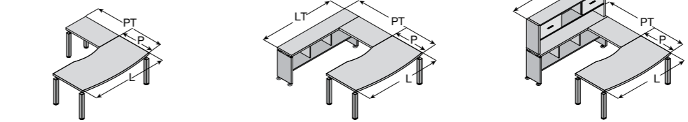
PT 200 x H 73,3 P 100 L 200 PT 241 x H 73,3 P 100 L 200 - LT 200 PT 241 x H 73,3 / 149,6 P 100 L 200 - LT 200
