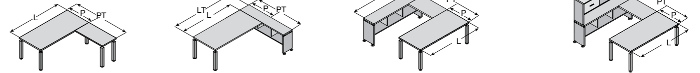
PT 190 x H 73,3 P 90 L 160 L 180 L 200 PT 200 x H 73,3 P 100 L 160 - LT 201 L 180 - LT 221 L 200 - LT 241 PT 231 x H 73,3 P 90 L 160 - LT 200 L 180 - LT 200 L 200 - LT 200 PT 231 x H 73,3 / 149,6 P 90 L 160 - LT 200 L 180 - LT 200 L 200 - LT 200
