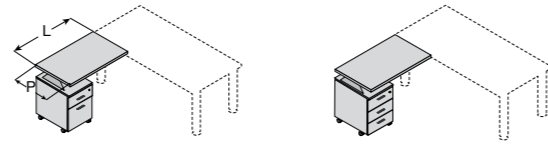
P 60 x H 73,3 L 100 P 60 x H 73,3 L 100
