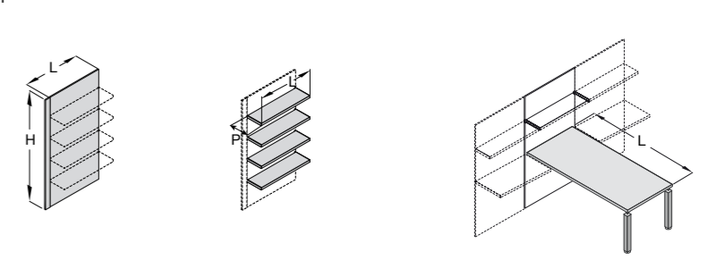
L 45 x H 161,5 L 60 L 90 L 45 x H 201,5 L 60 L 90 L 45,1 x P 27 x H 3,8 L 60,1 L 90,1 L 45,1 x P 49 x H 3,8 L 60,1 L 90,1 P 90 x H 74 L 160 L 180 L 200
